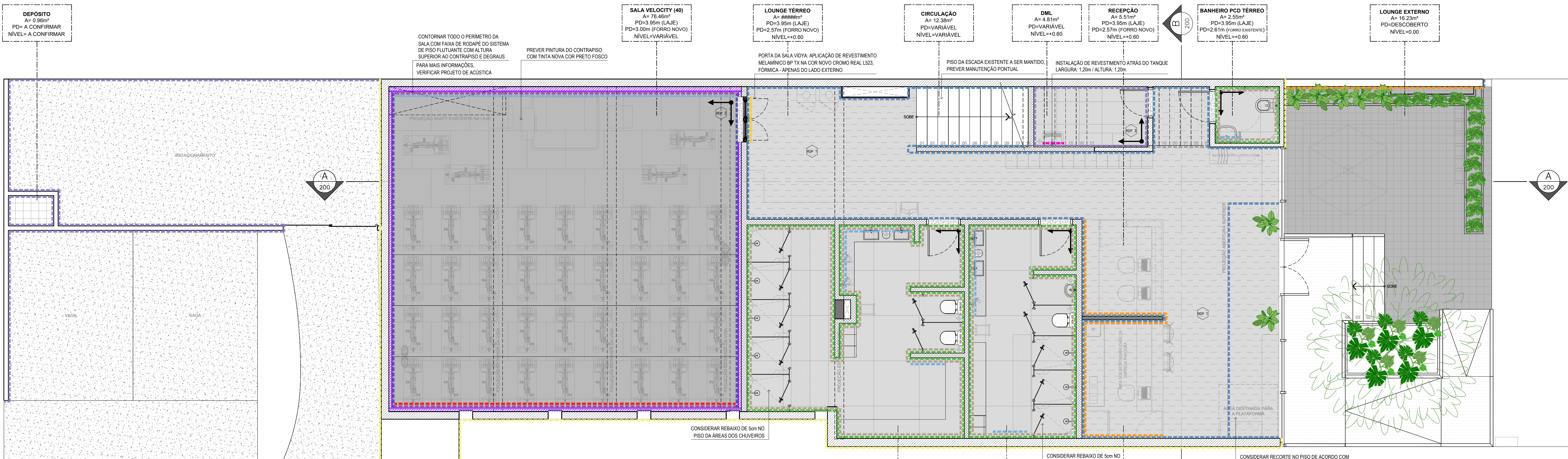
PLANTA ACABAMENTOS TÊRREO ESCALA 1:50
