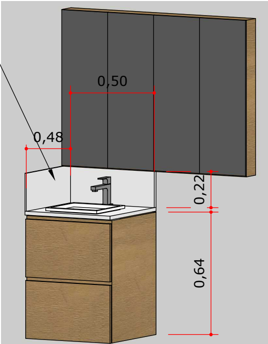
A :: PERSPECTIVA W.C 2 000 Escala: 1:20
