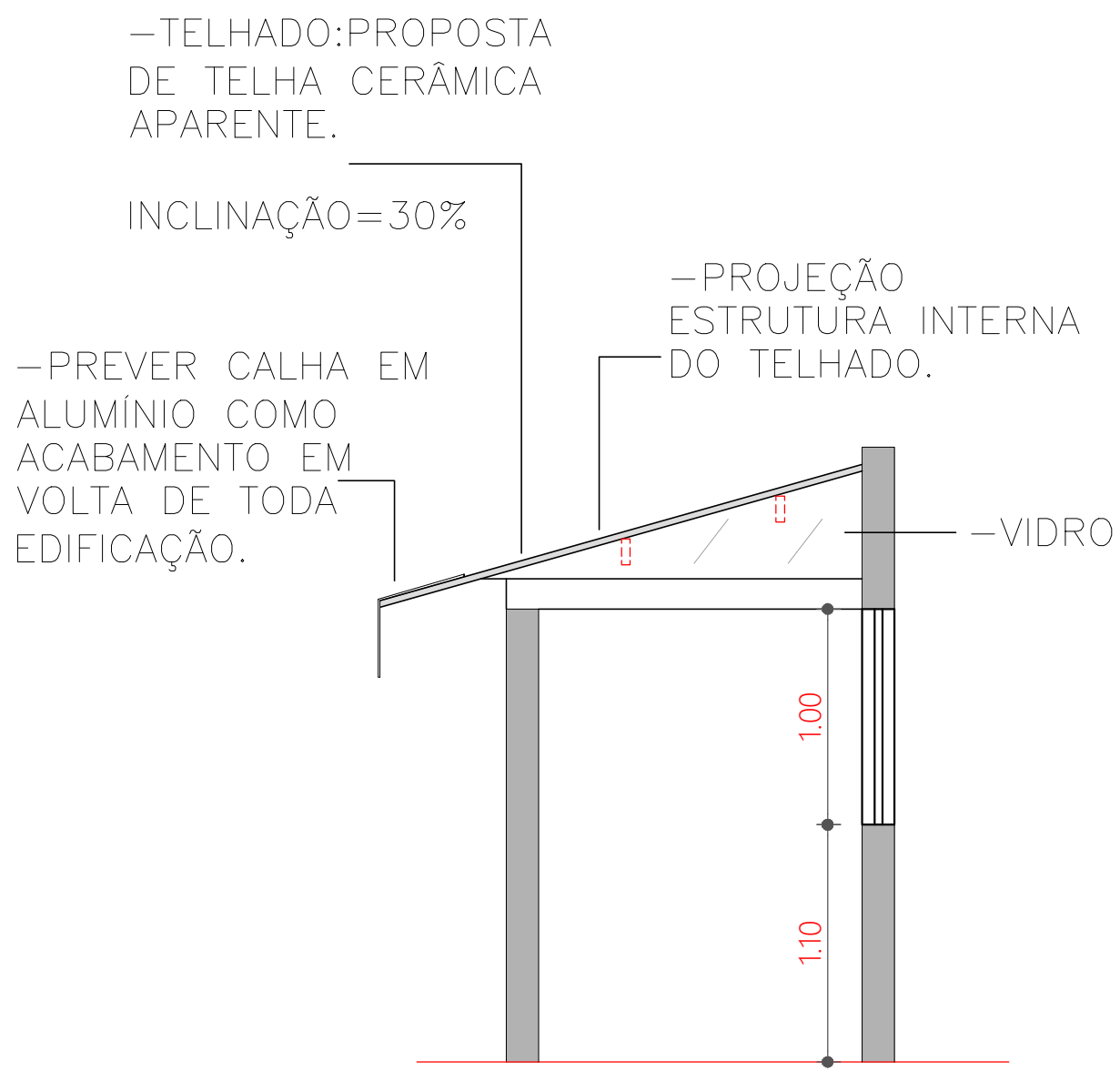
CORTE AA
