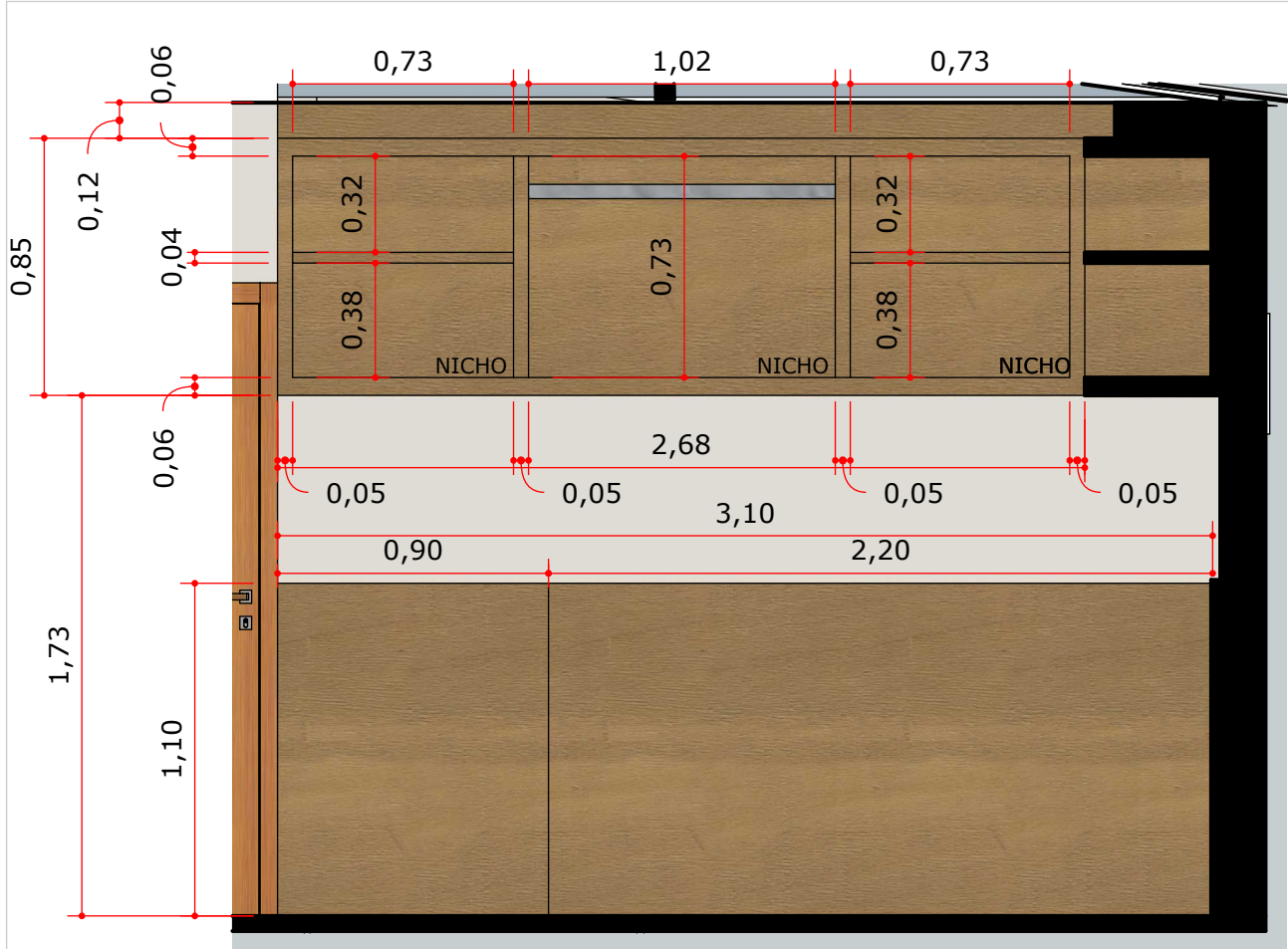
A :: VISTA 05- DORMITÓRIO 1 000 Escala: 1:25
