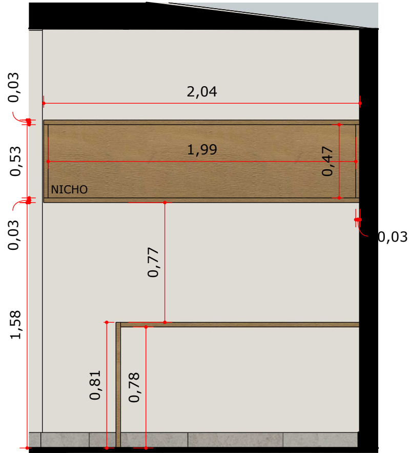
A :: VISTA 03- SUÍTE 000 Escala: 1:25
