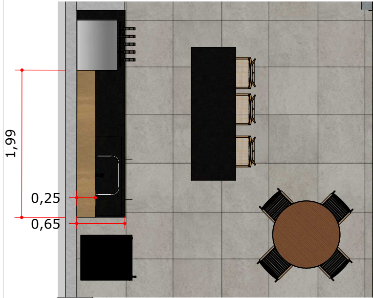
A :: VISTA SUPERIOR ÁREA GOURMET
