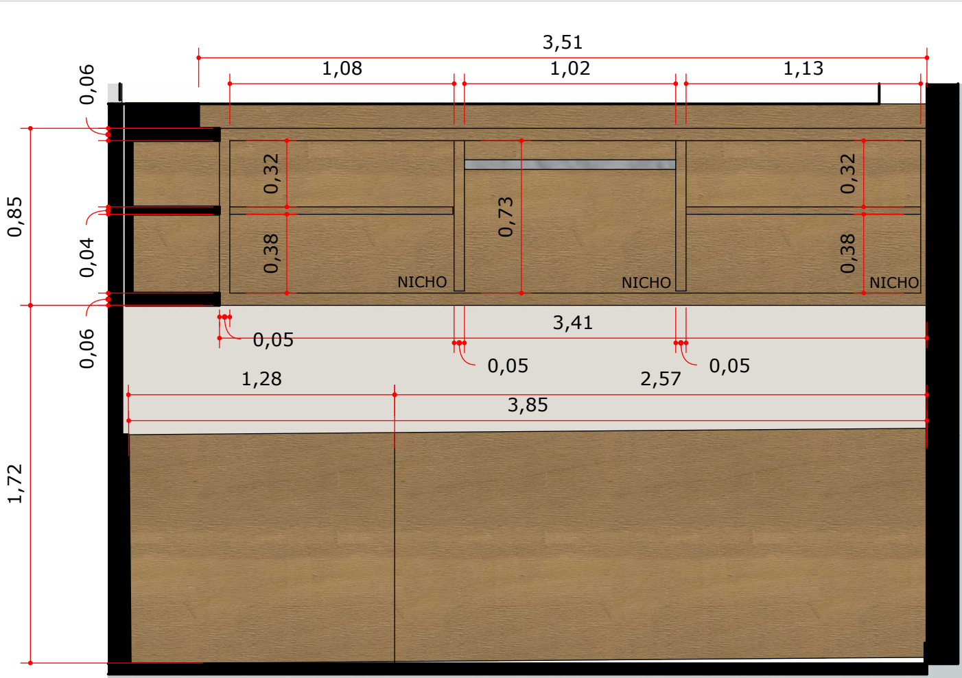
A :: VISTA 06 - DORMITÓRIO 1 000 Escala: 1:25
