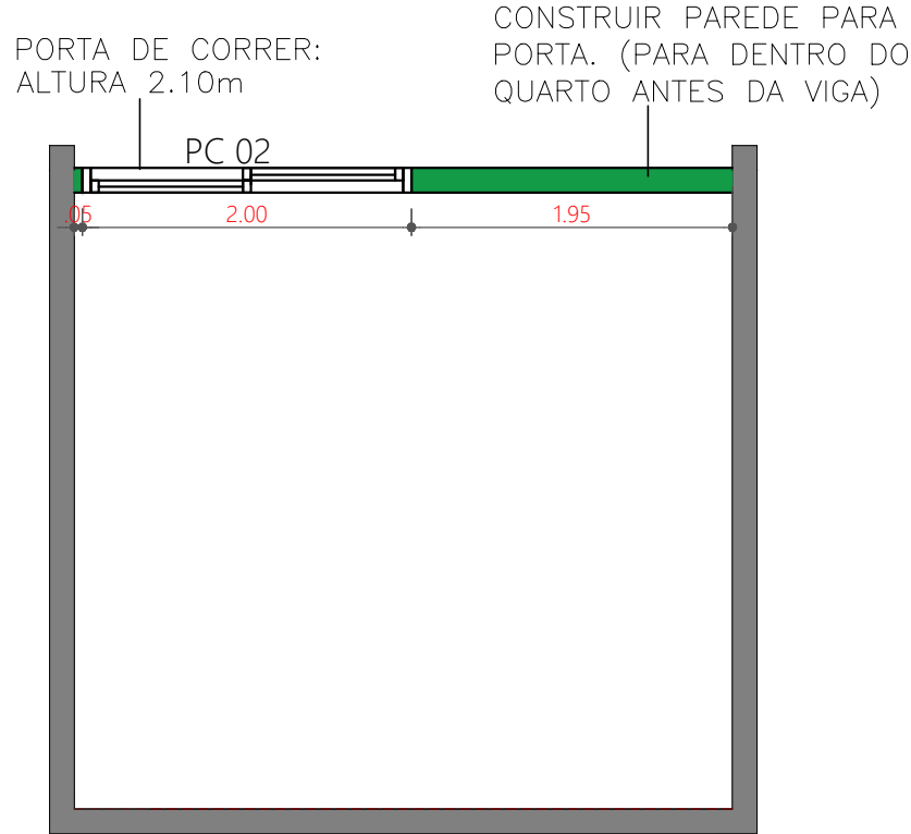
PLANTA-QUARTINHO
