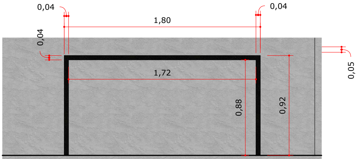
A :: VISTA 2 - ÁREA GOURMET 000 Escala: 1:20
