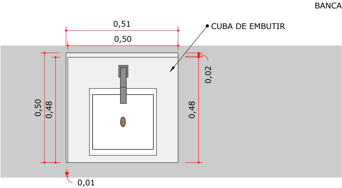
A :: VISTA SUPERIOR W.C 2 000 Escala: 1:10
