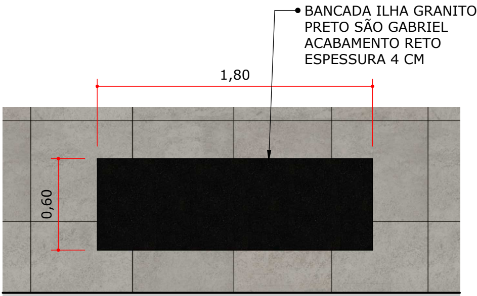
A :: VISTA SUPERIOR ÁREA GOURMET 000 Escala: 1:25
