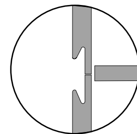
DET.03 PUXADOR CAVA LATERAL
