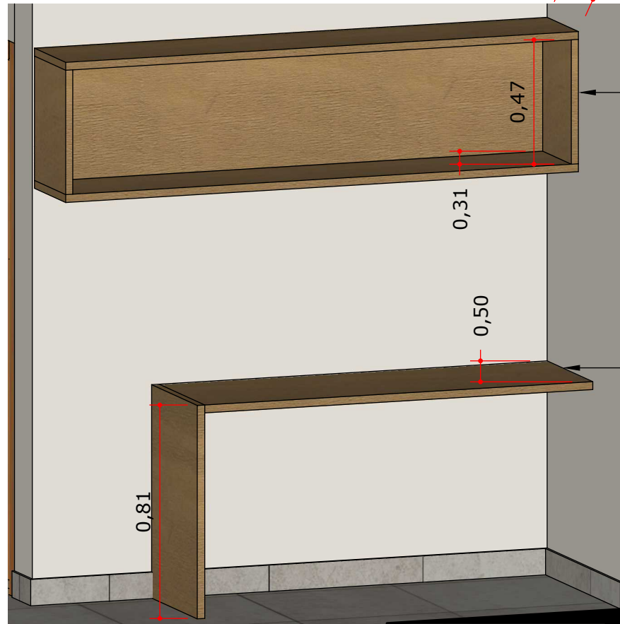
A :: PERSPECTIVA-SUÍTE 000 Escala: 1:20
