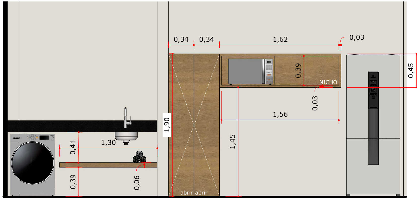
A :: VISTA 02 - LAVANDERIA E COZINHA 000 Escala: 1:25
