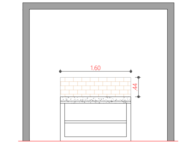
DETALHAMENTO REVESTIMENTO COZINHA
