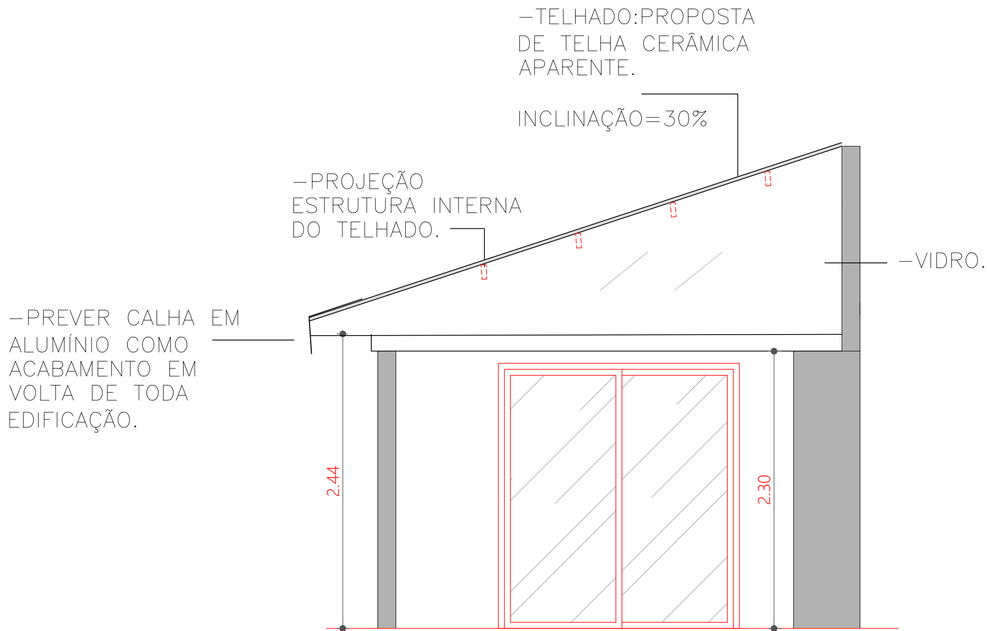
ELEVAÇÃO 01
