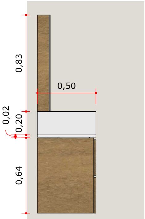
A :: VISTA LATERAL W.C 2 000 Escala: 1:20
