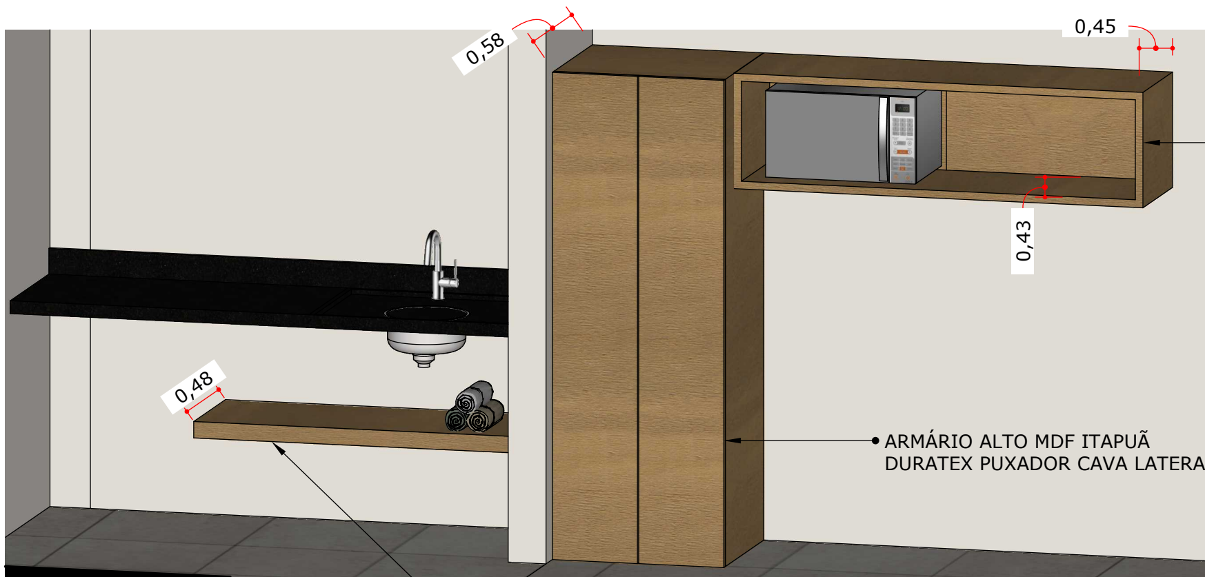
A :: PERSPECTIVA- LAVANDERIA E COZINHA 000 Escala: 1:20
