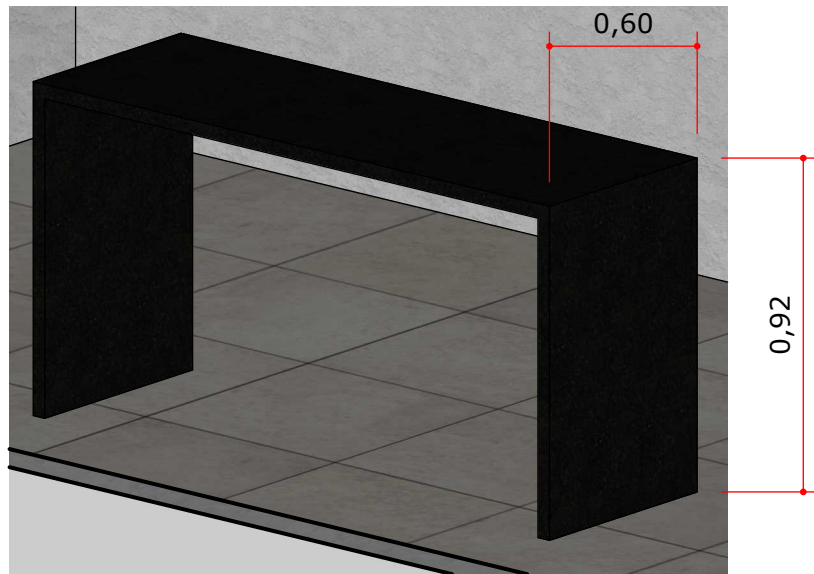
A :: PERSPECTIVA ÁREA GOURMET 000 Escala: 1:20
