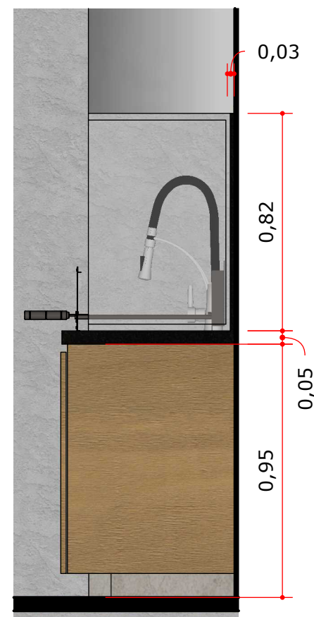
A :: VISTA LATERAL- ÁREA GOURMET 000 Escala: 1:20
