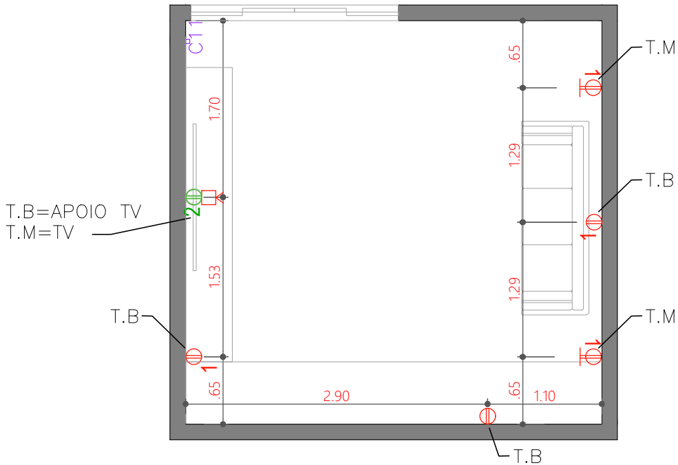
PLANTA-QUARTINHO
