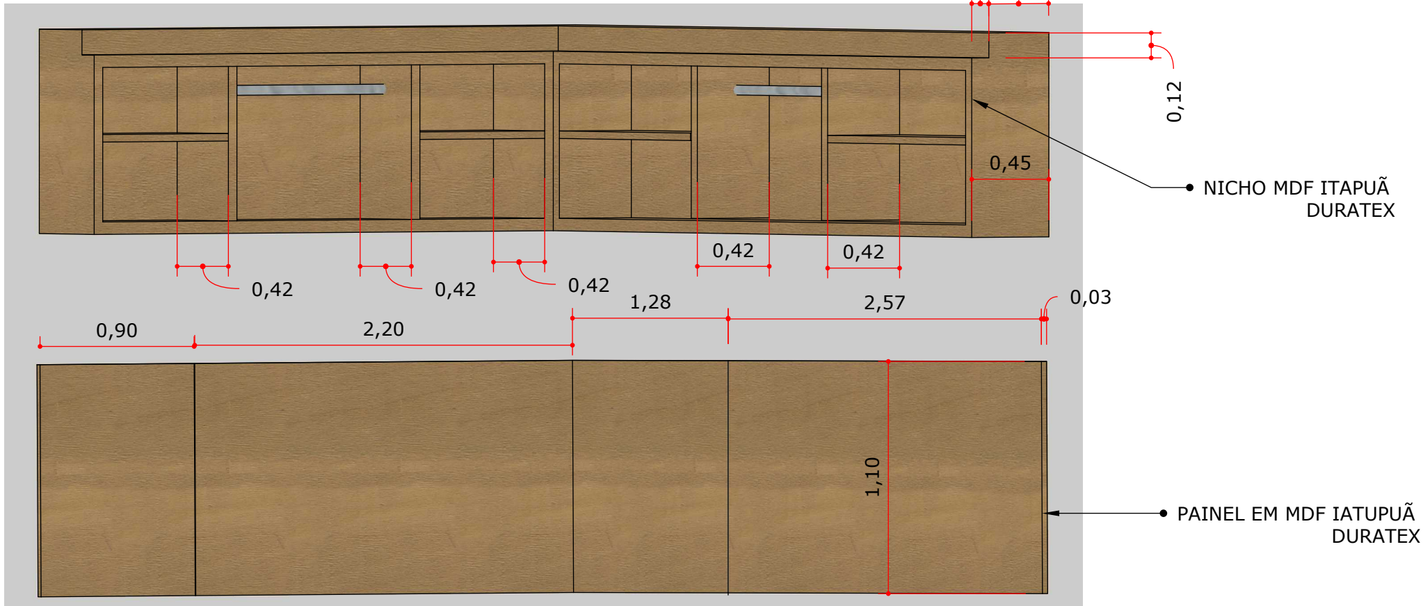
A :: PERSPECTIVA 000 Escala: 1:25
