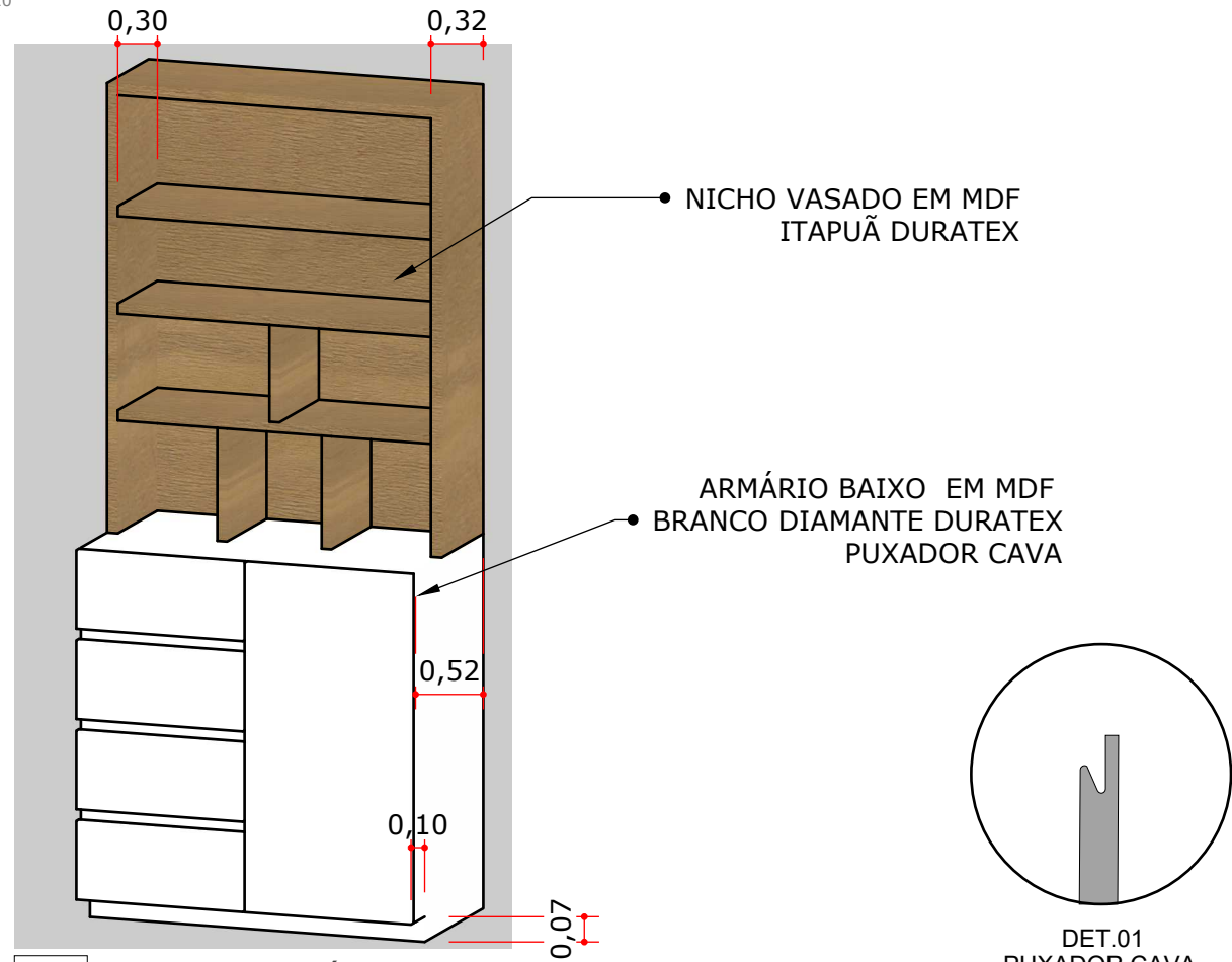
A :: PERSPECTIVA-SUÍTE 000 Escala: 1:20
