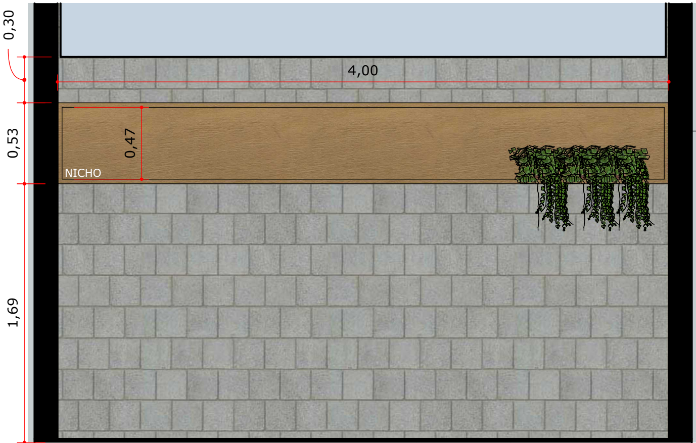
A :: VISTA 06 - DORMITÓRIO 2 000 Escala: 1:25
