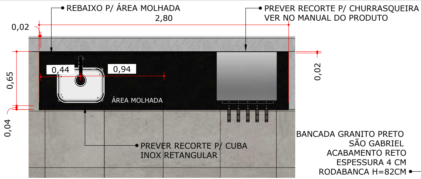
A :: VISTA SUPERIOR ÁREA GOURMET 000 Escala: 1:50
