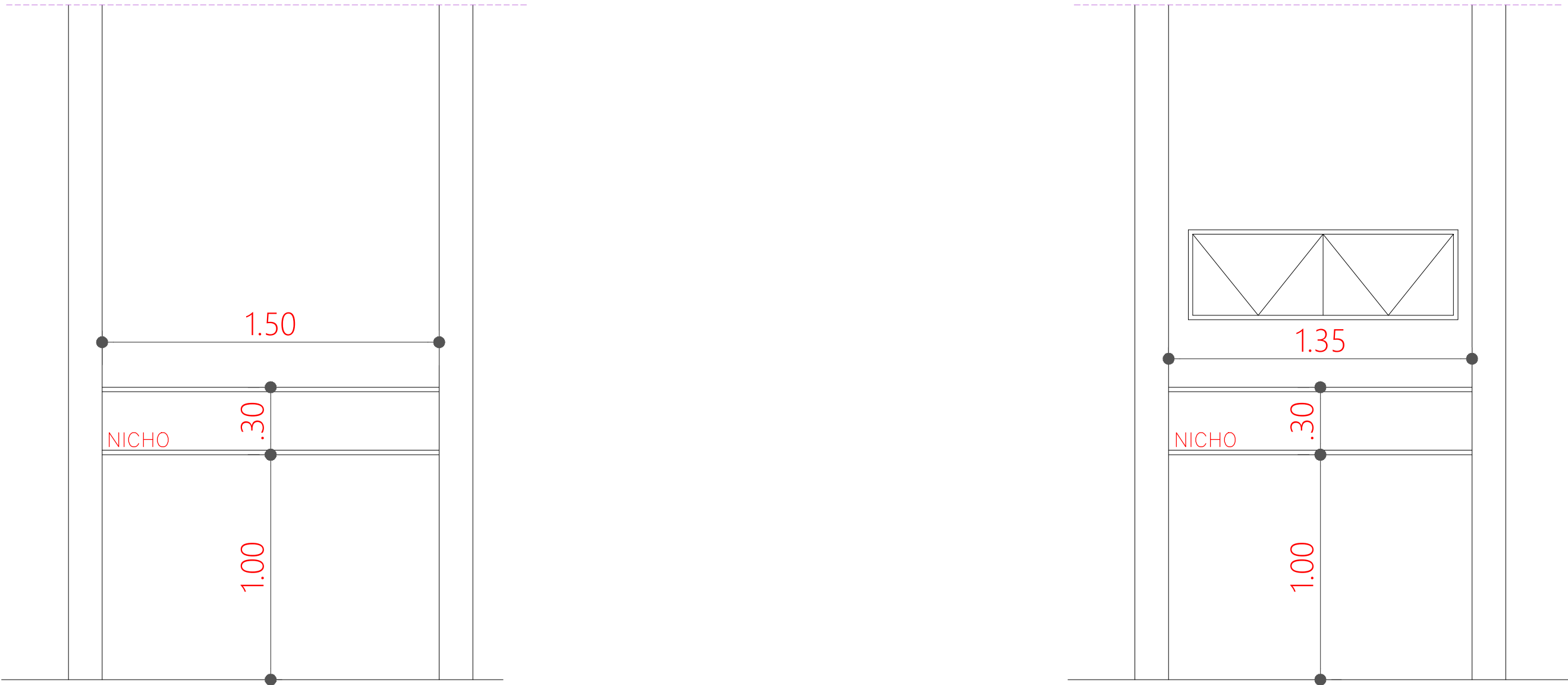
DETALHAMENTO 01- BANHEIRO SUITE
