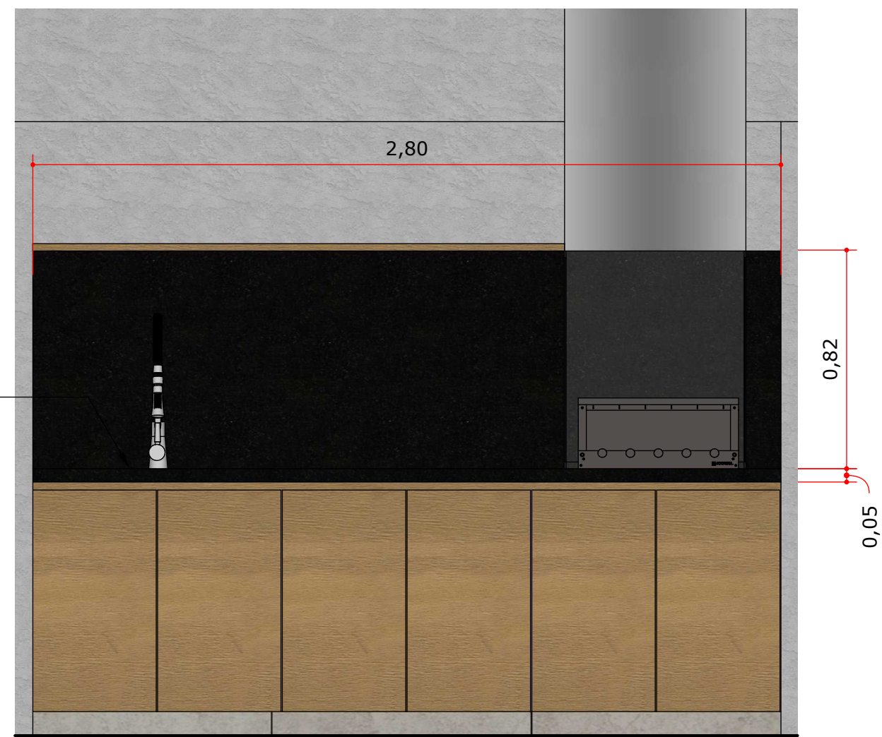
A :: VISTA 1 - ÁREA GOURMET 000 Escala: 1:20
