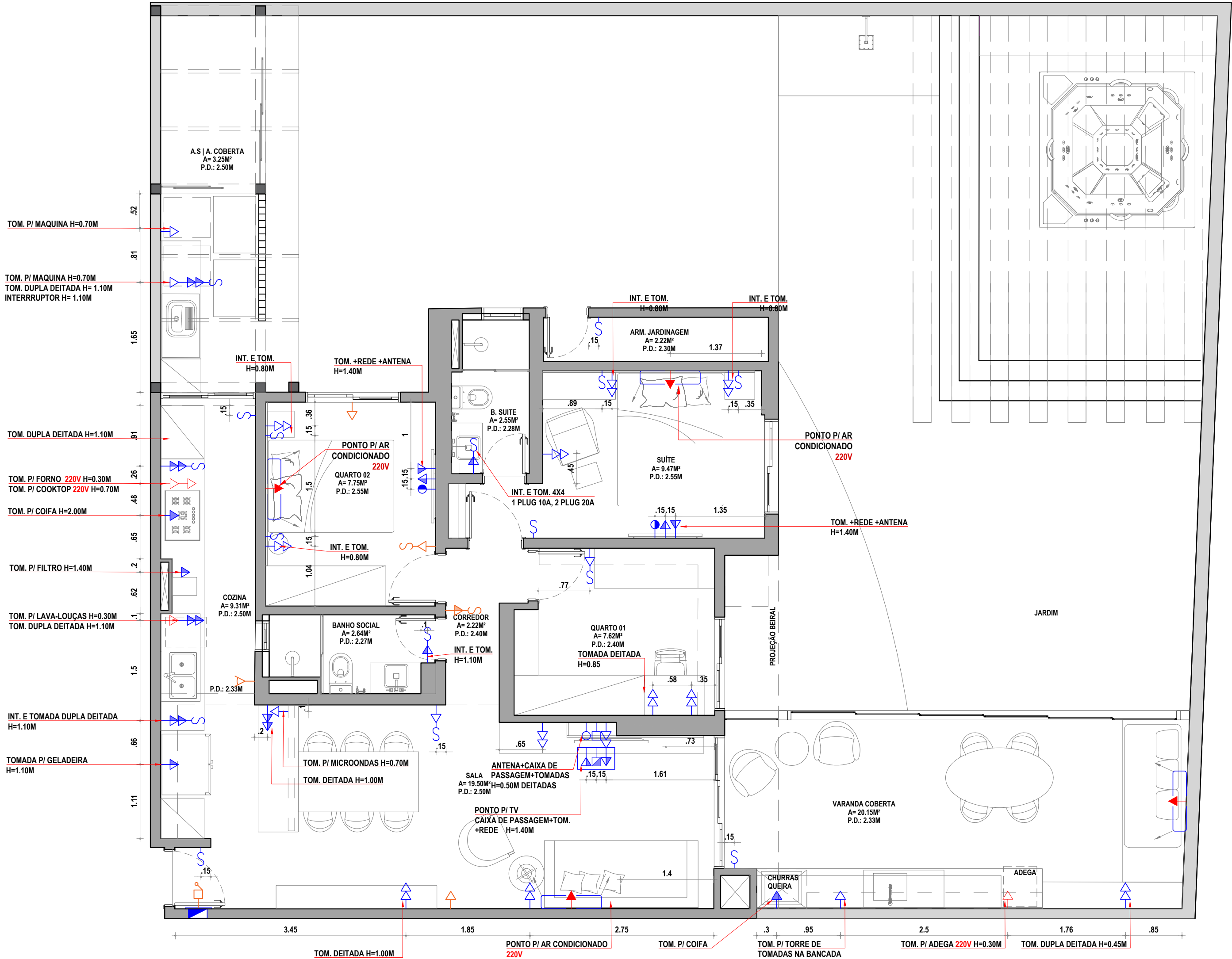
01 PLANTA DE ELÉTRICA ESCALA: 1/50
